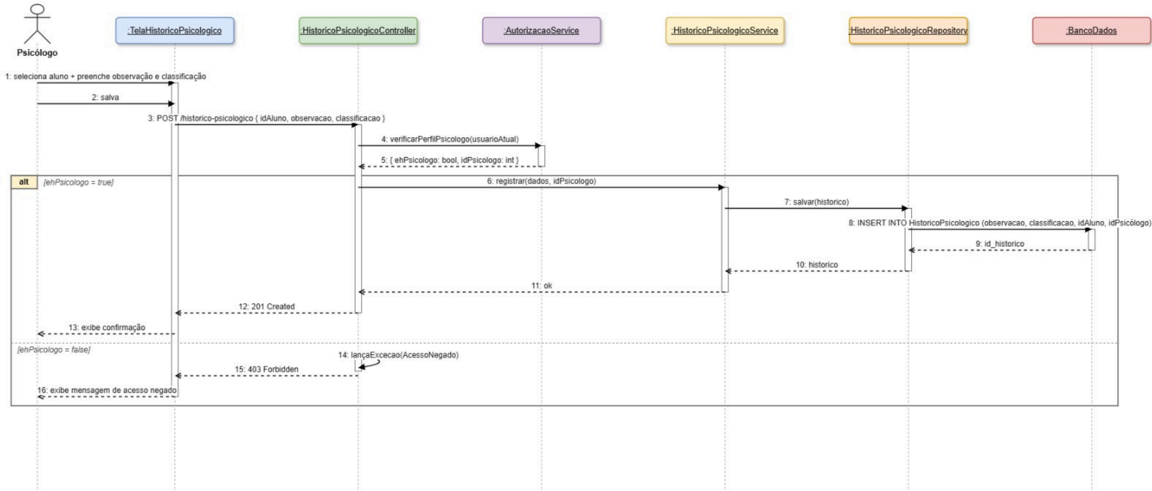
Diagrama de Sequência - UC-22 Manter registros de saúde mental
